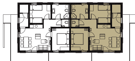
tloris etaže
